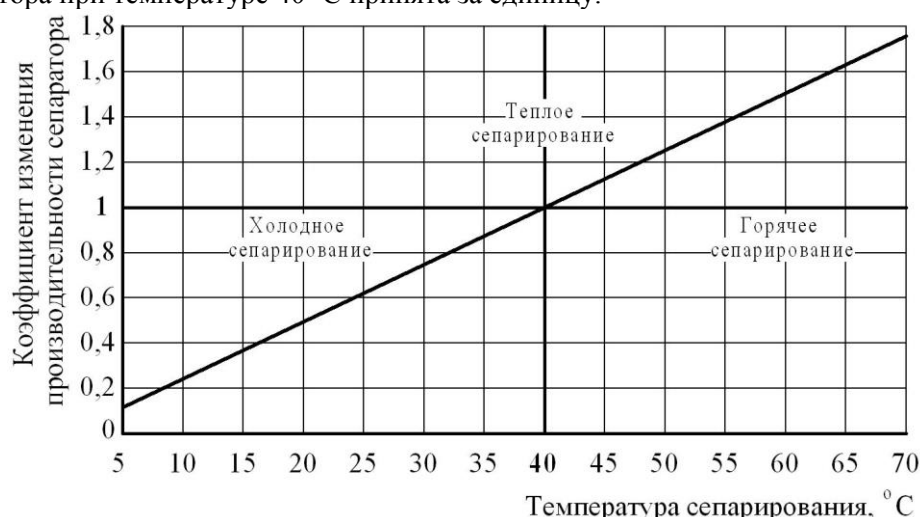
Рис. 1. Изменение производительности сепаратора-сливкоотделителя в зависимости от температуры сепарирования
