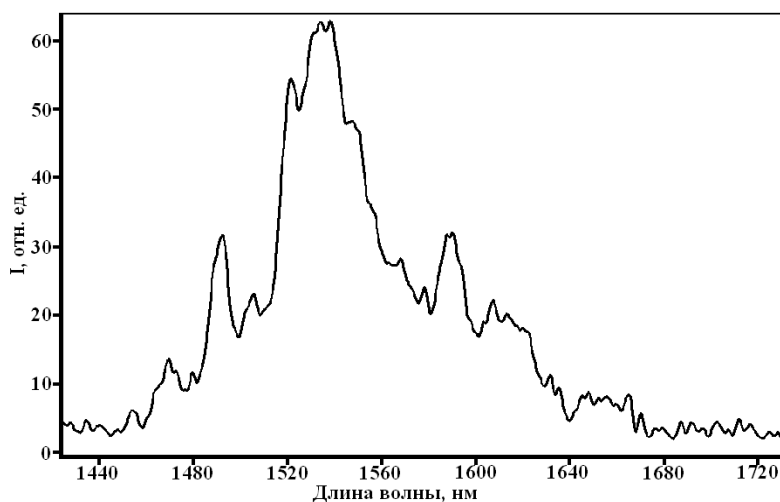
Рис. 1. Спектр стоксовой ИК-люминесценции твердых растворов Y_{0.84-x}Yb_{0.15}Er_{0.01}Tm_xAl_3(BO_3)_4 в области 1500 нм при возбуждении излучением с длиной волны в диапазоне 940–980 нм
