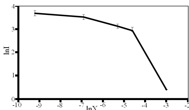
Рис. 2. Логарифмическая зависимость интенсивности стоксовой ИК-люминесценции твердых растворов \text{Y}_{0,84-x}\text{Yb}_{0,15}\text{Er}_{0,01}\text{Tm}_x\text{Al}_3(\text{BO}_3)_4 в области 1500 нм от концентрации ионов тулия при возбуждении излучением с длиной волны в диапазоне 940–980 нм
