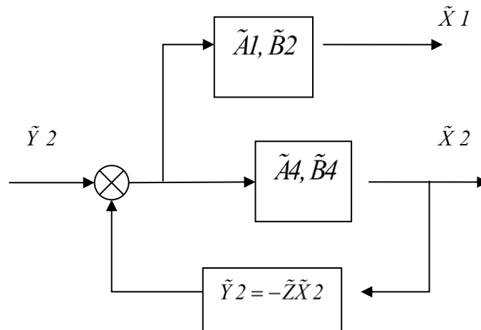
Рис. 2. Соединение подсистем с обратной связью.
