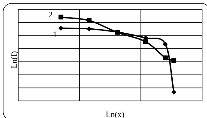
Рис. 6. Логарифмические зависимости интенсивности люминесценции в полосах 1) 1036 нм; 2) 1652 нм в твердом растворе (Y_{0,85-x}Yb_{0,1}Er_{0,05}Ho_x)_3Al_5O_{12} от концентрации ионов Ho^{3+}
