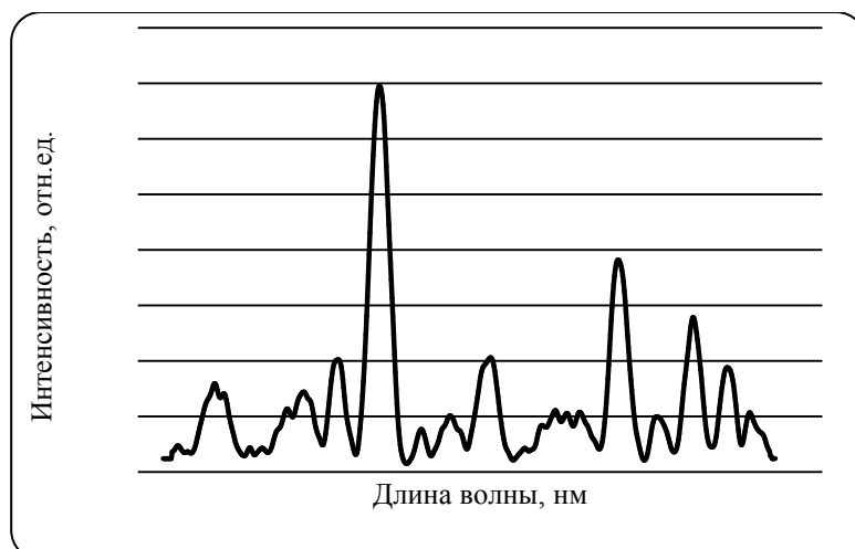
Рис. 3. Фрагмент спектра стоксовой ИК-люминесценции твердых растворов (Y_{0,85-x}Yb_{0,1}Er_{0,05}Ho_x)_3Al_5O_{12} в области 1440–1680 нм при возбуждении лазерным излучением с длиной волны 940 нм
