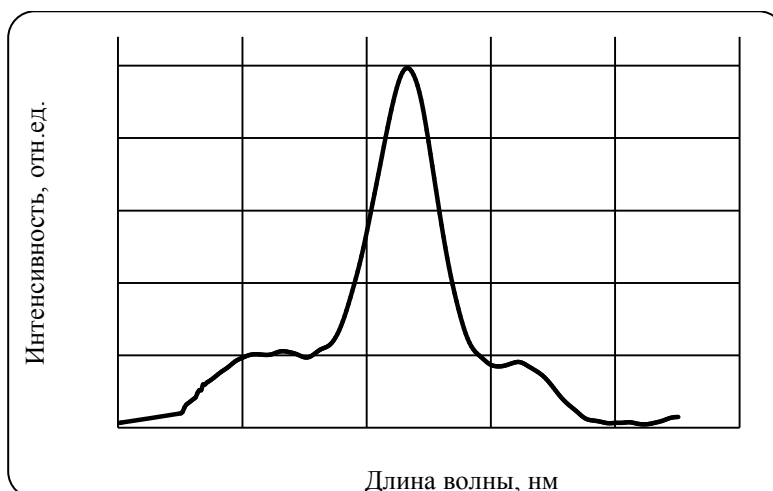
Рис. 2. Фрагмент спектра стоксовой ИК-люминесценции твердых растворов (Y_{0,85-x}Yb_{0,1}Er_{0,05}Ho_x)_3Al_5O_{12} в области 990–1070 нм при возбуждении лазерным излучением с длиной волны 940 нм
