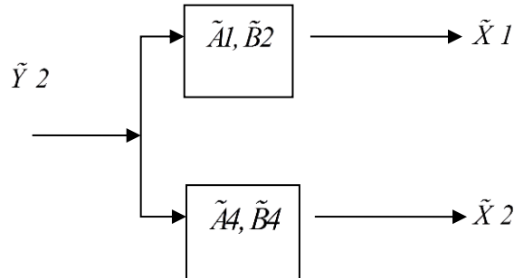
Рис. 1. Параллельное соединение двух подсистем.
