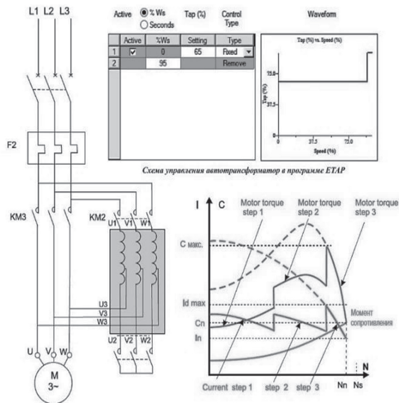
Рис. 8. Схема пуска асинхронного двигателя через автотрансформатор
